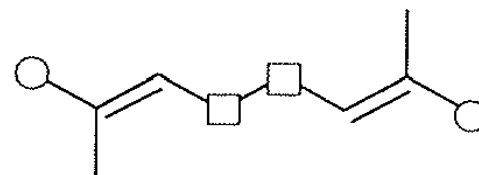
spojení "pata - pata"
