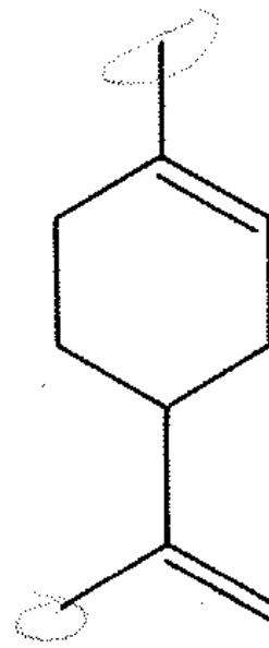
zjednodušený vzorec limonenu
