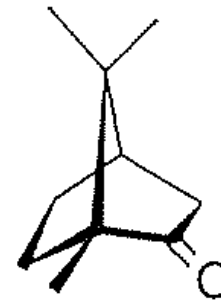
kafr
