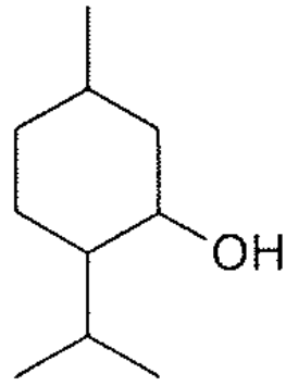
menthol
