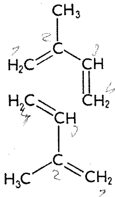
dvě molekuly isoprenu
