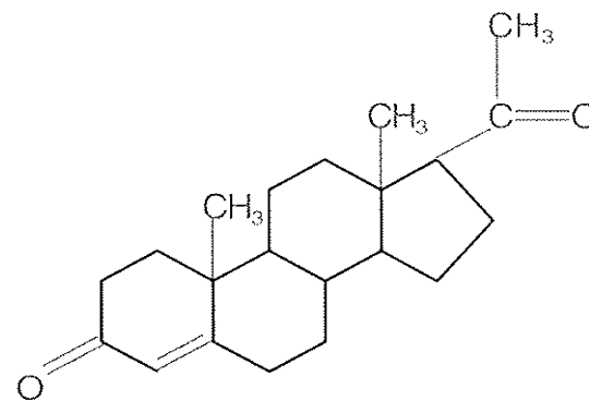
progesteron
