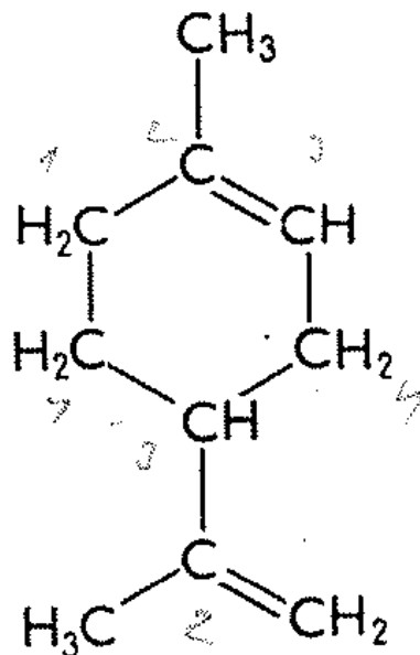
limonen
