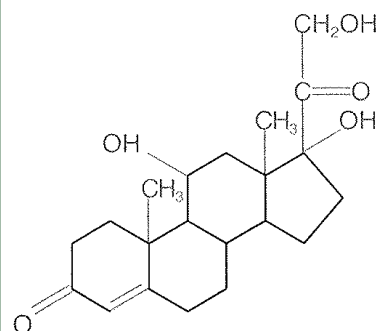
kortisol
