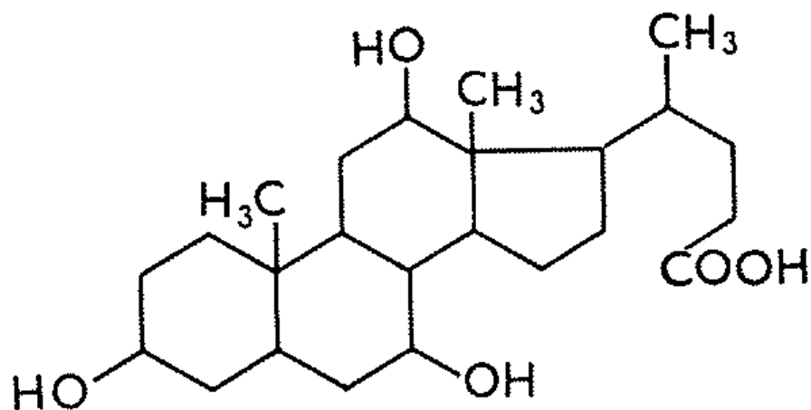
kyselina cholová
