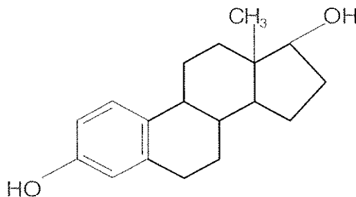
estradiol
