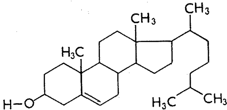
cholesterol volný
