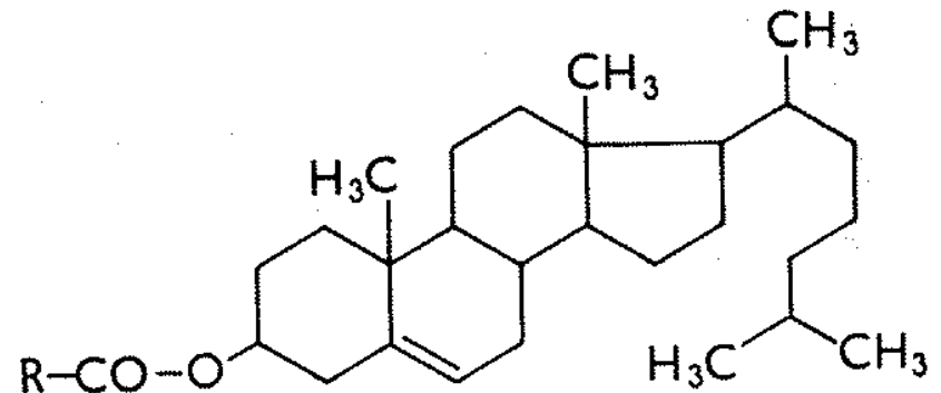
cholesterol esterifikovaný (acylcholesterol)
