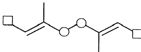
spojení "hlava - hlava"
