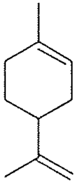
limonen
