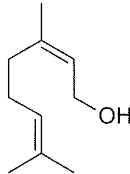
geraniol
