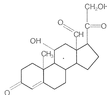
aldosteron
